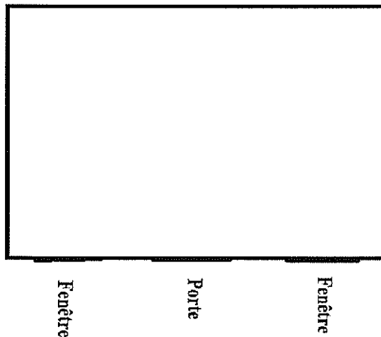
Figure 2 : Bâtiment modulaire pour presses et essais mécaniques 6m x 3m, H : 2,6m
